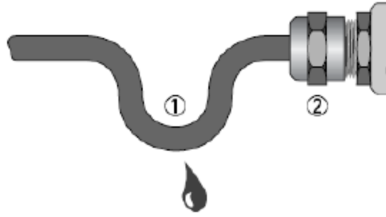
Рисунок 4 – Правила прокладки и присоединения кабеля в соответствии со степенью защиты IP66/ IP67/ IP68
