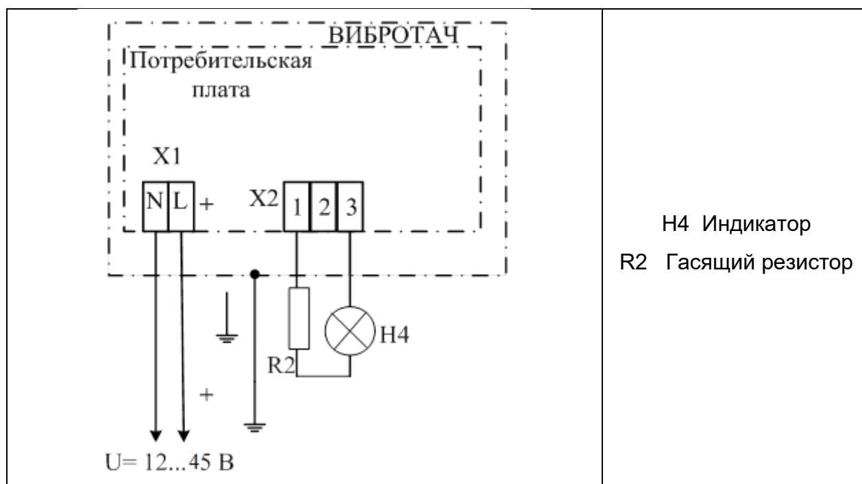
Рисунок 6.3 – Схема подключений для проверки функционирования сигнализаторов исполнения 52
